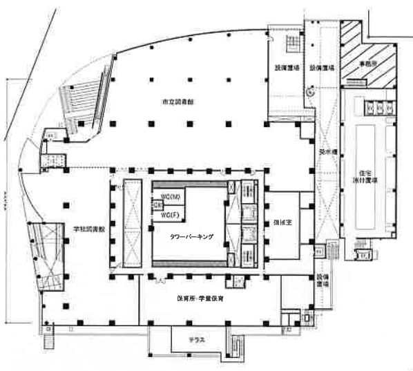
複合施設全体2階平面図
