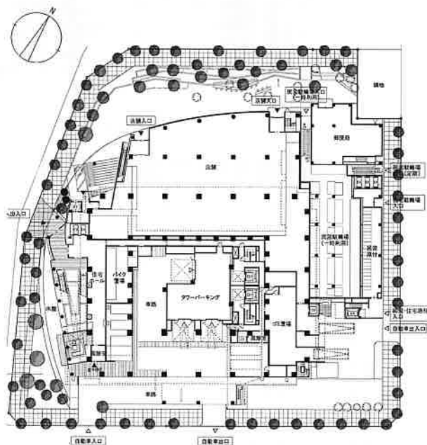
複合施設全体1階平面図
